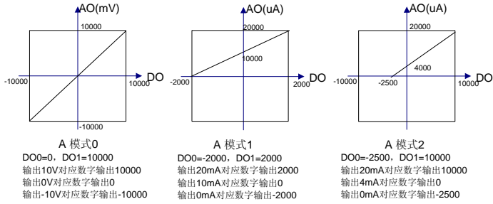
图 5-3 特性更改举例
