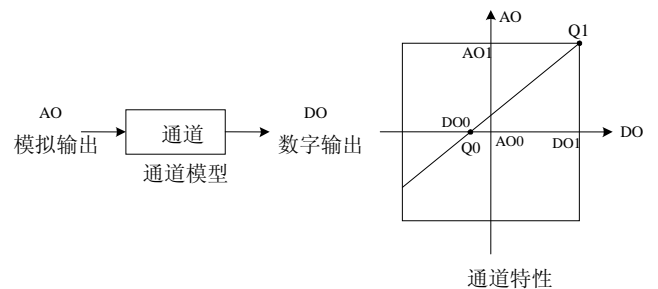
图 5-1 MC100-4DA/2DA 的通道特性示意图
