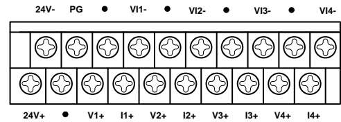
图 4-1 MC-4DA 端子图
