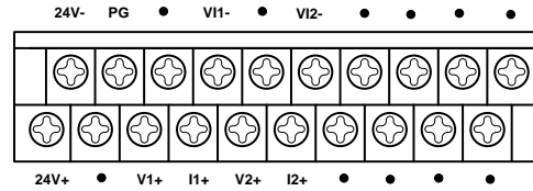
图 4-2 MC-2DA 端子图
