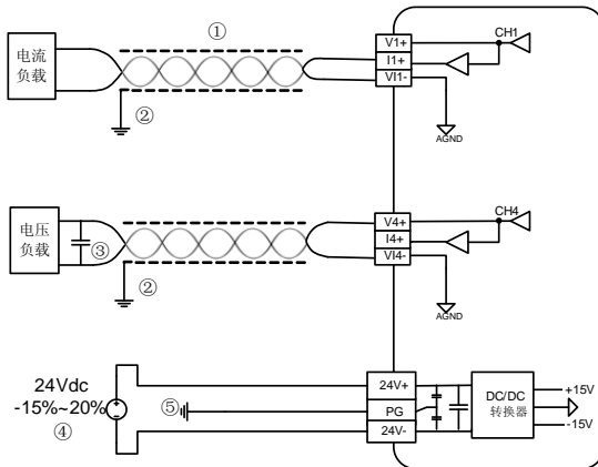
图 2-5 MC100-4DA/2DA 用户端子布线示意图
