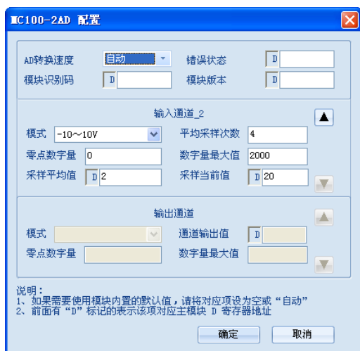
图 6-3 设置各通道特性 2
