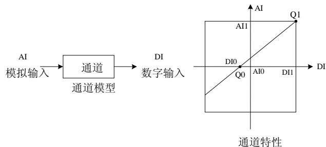
图 5-1 MC100-2AD 的通道特性示意图
