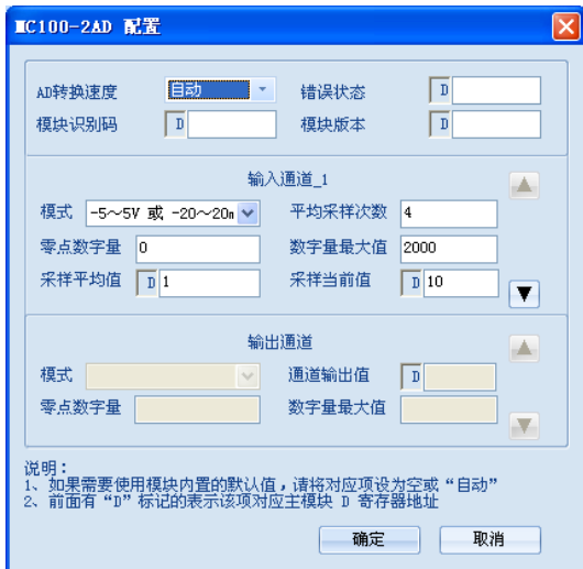
图 6-2 设置各通道特性 1
