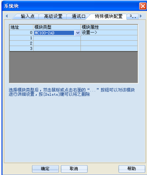
图 6-1 设置 MC100-2AD 模块属性
