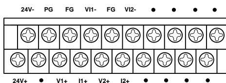
图 4-1 MC100-2AD 模拟量输入模块用户端子图
