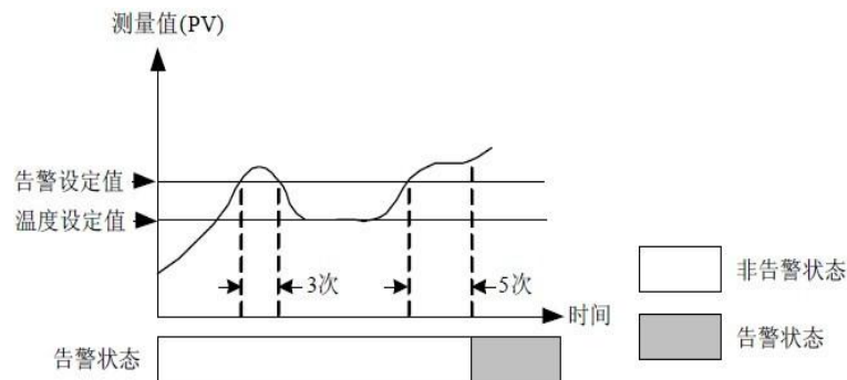
图 4-28 告警延迟次数示意图
