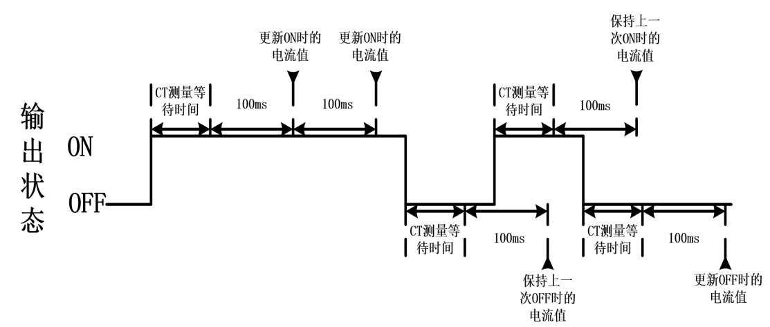
图 4-29 CT 更新时间
