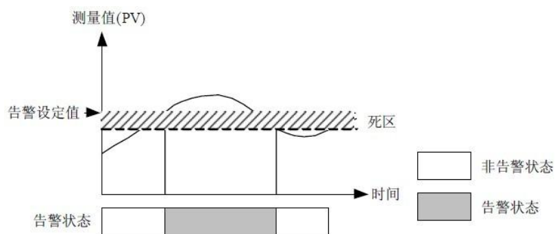
图 4-25 上限输入值和偏差上限告警示意图
