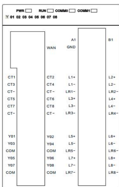
图 1-3 MTCW-08-CT 用户端子图
