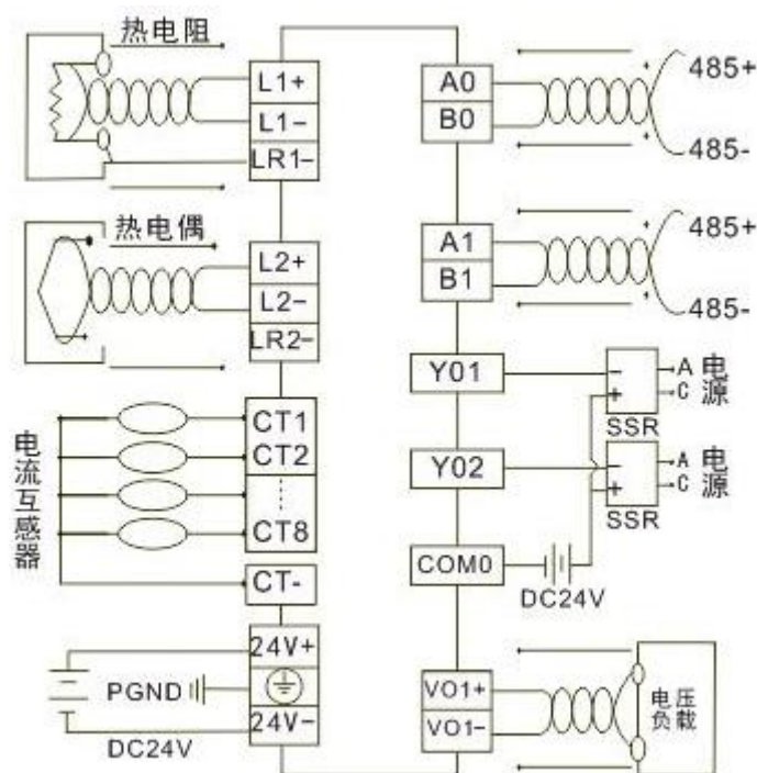
图 2-4 MTCW 输入用户端子布线示意图
