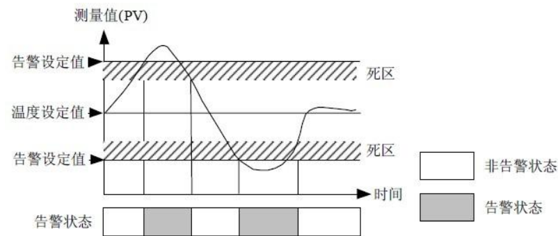
图 4-27 偏差上/下限告警示意图
