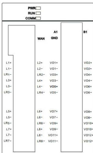
图 1-5 MTCW-08-NV 用户端子图
