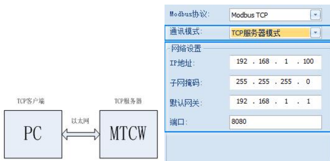
图 3-3 TCP 服务器配置
