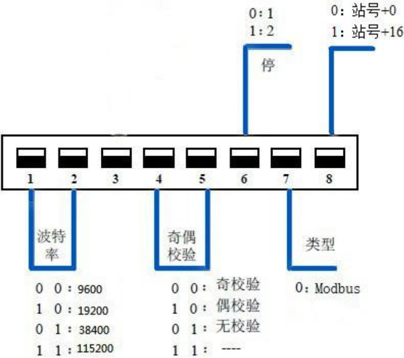
图 3-1 拨码开关说明
