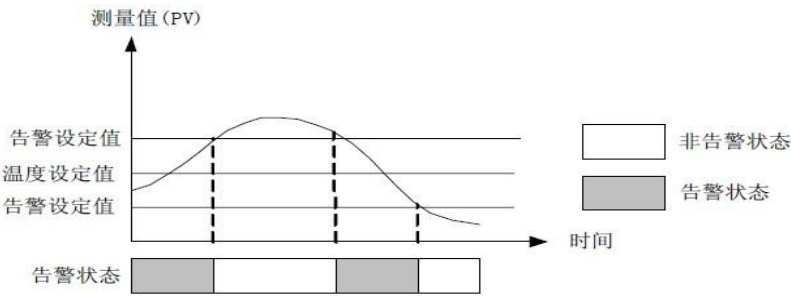
图 4-21 范围告警示意图
