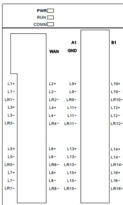
图 1-7 MTCW-16-NN 用户端子图
