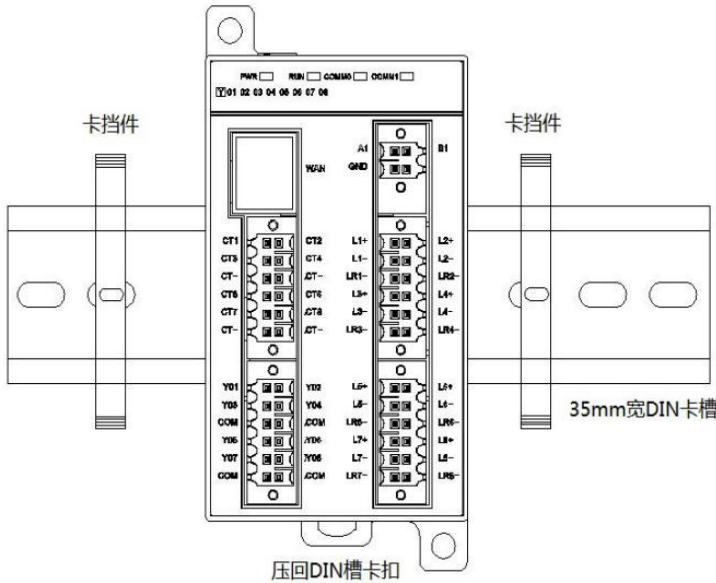
图 2-2 采用 DIN 槽安装固定
