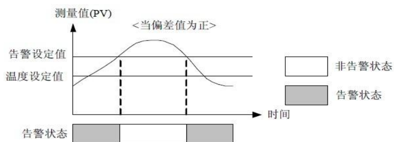
图 4-18 偏差下限告警示意图 (偏差值为正)
