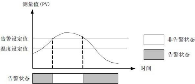
图 4-22 不带等待的偏差下限示意图
