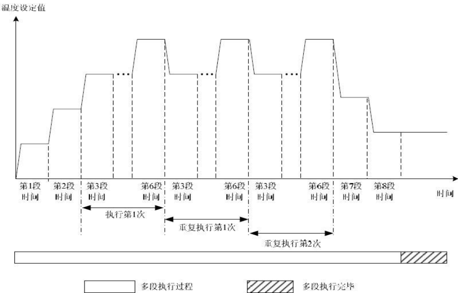
图 4-10 多段设定值执行示意图
