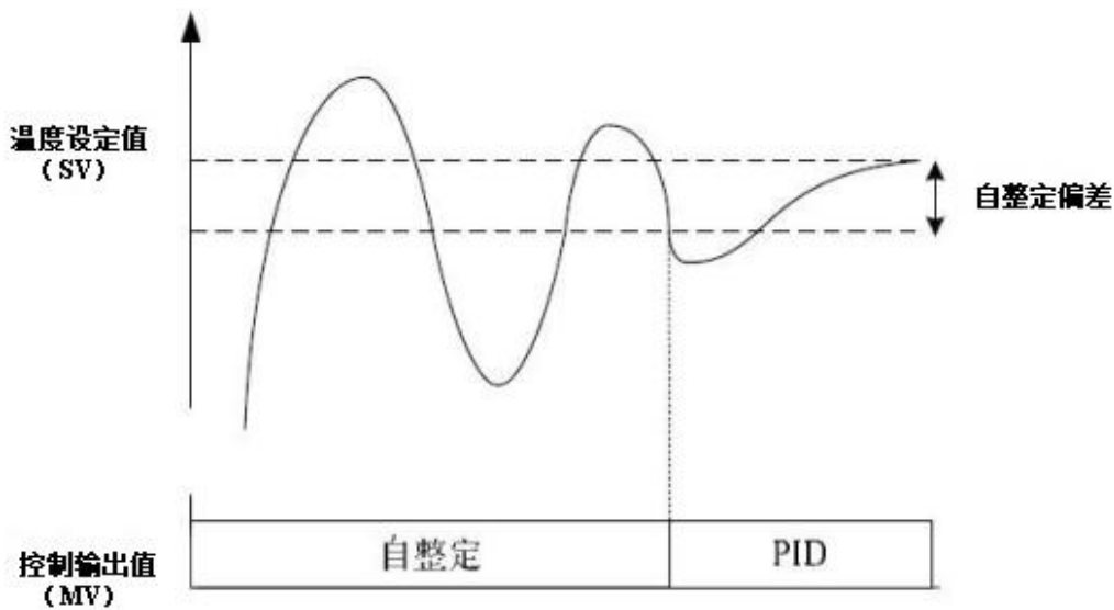
图 4-5 自整定
