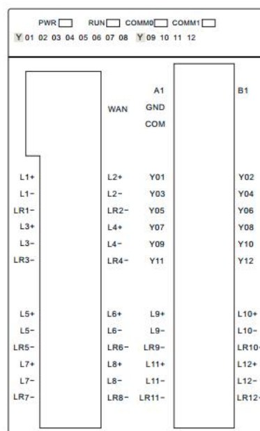
图 1-6 MTCW-12-NT 用户端子图
