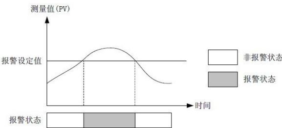
图 4-14 上限输入值告警示意图
