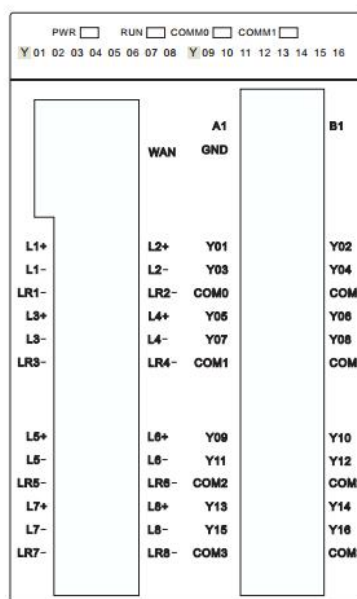
图 1-4 MTCW-08-NTT 用户端子图
