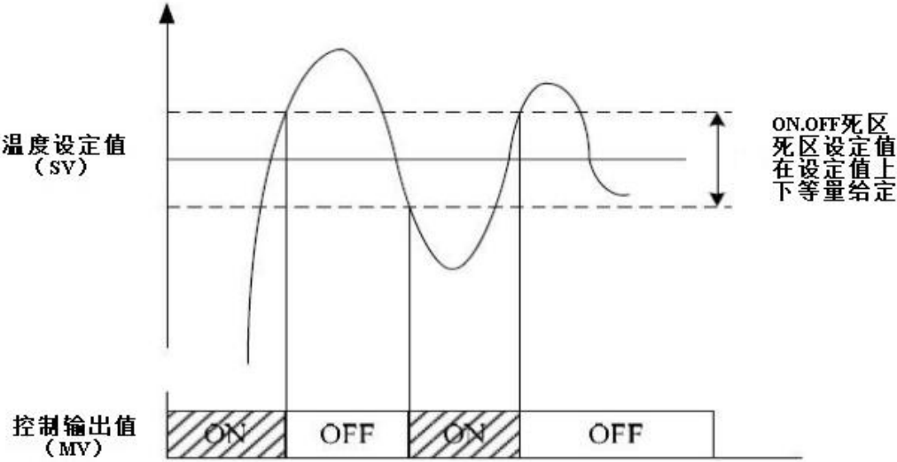
图 4-3 ON/OFF 控制
