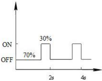
图 4-2 手动输出
