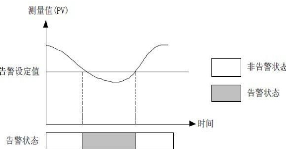
图 4-15 下限输入值告警示意图
